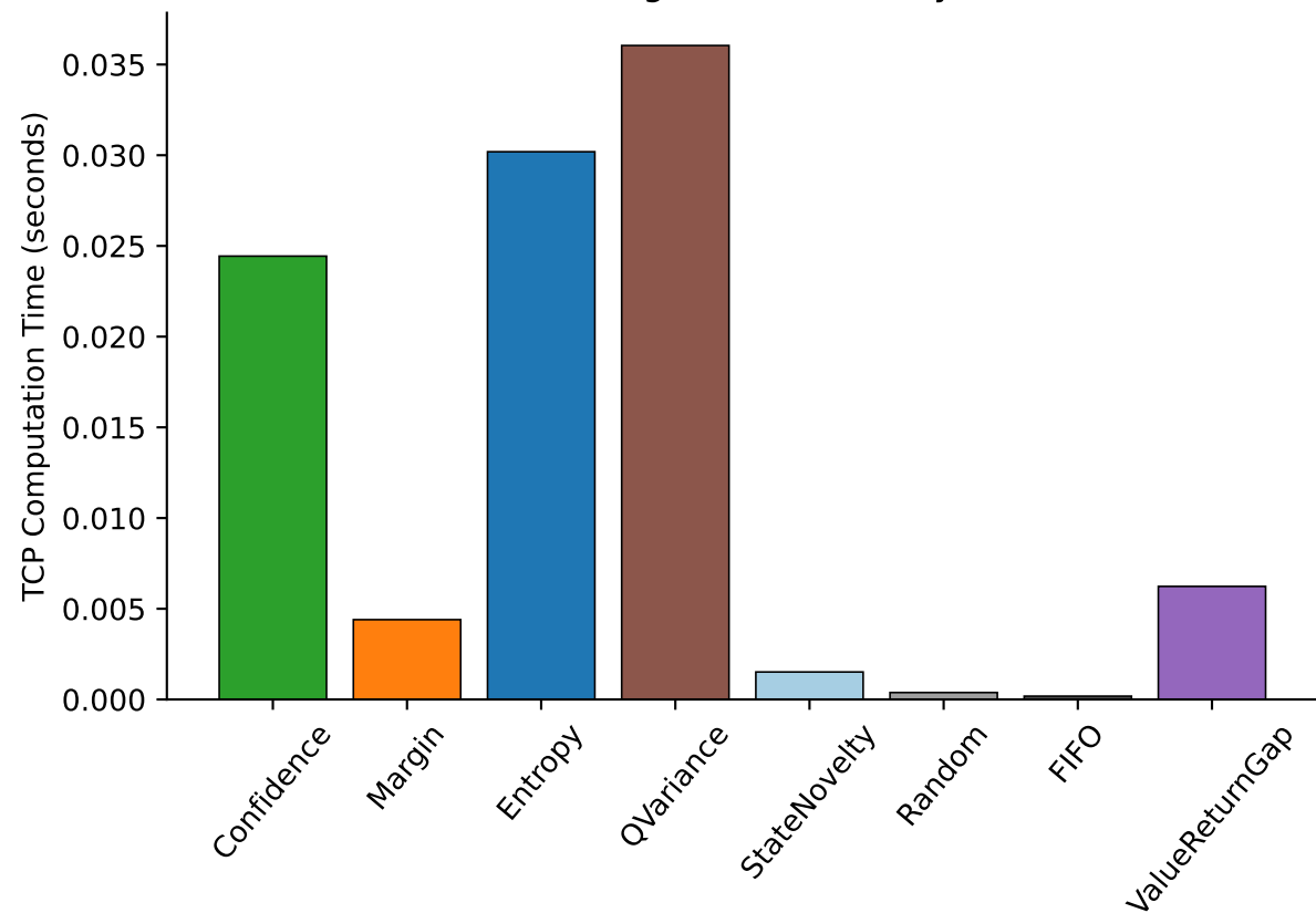
TCP Ranking Cost — Taxi (DynaQ)
